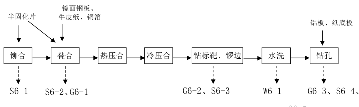
图 2.2-6 内层压合、钻孔工艺流程图
